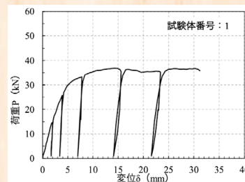
強度試験状況(上)と得られた荷重-変位曲線(右)の例(105×240mm) (25ER018号 評価書より抜粋)
