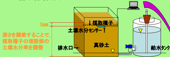
図3 作製した「種子の箱舟」
